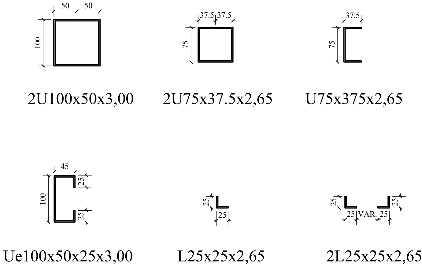
DETALHES DE PERFIS ESTRUTURAIS
