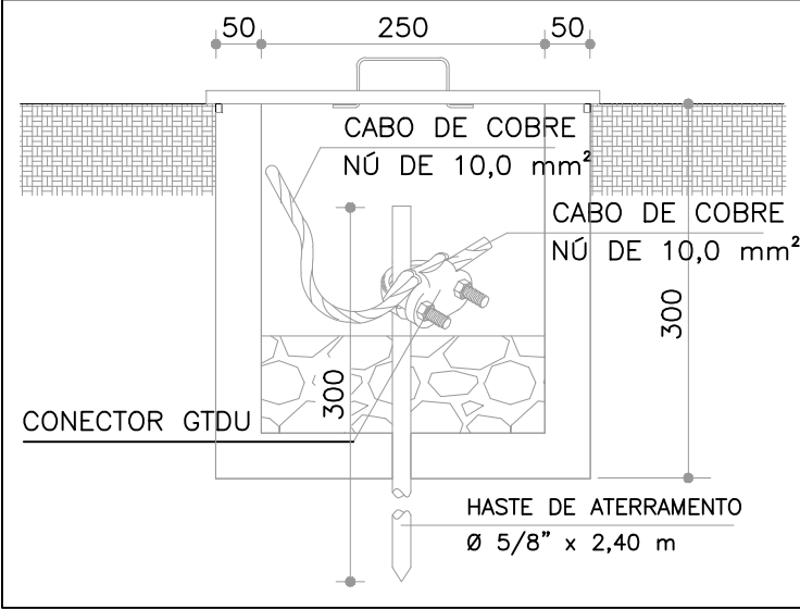
DETALHE CX. DE ATERRAMENTO SEM ESCALA
