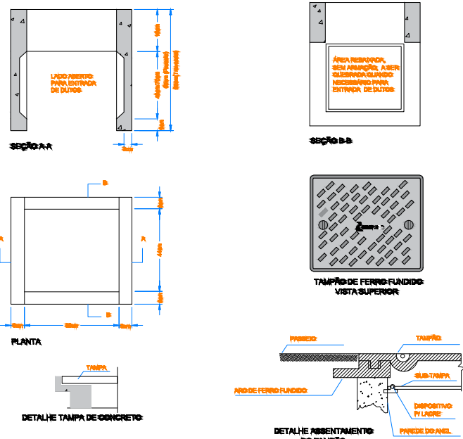
(Caixa de Passagem Tipo CP - 01)
